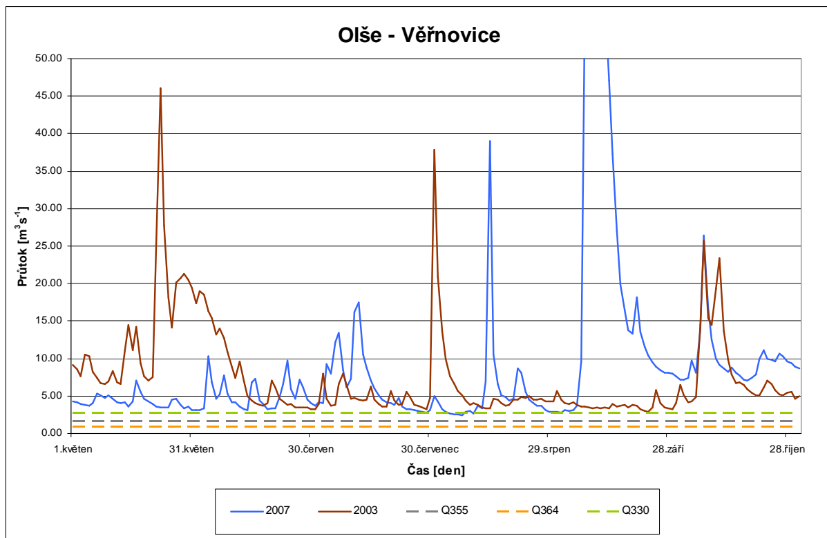
Hydrogramy vybraných povodňových událostí ve stanici Věřovice
