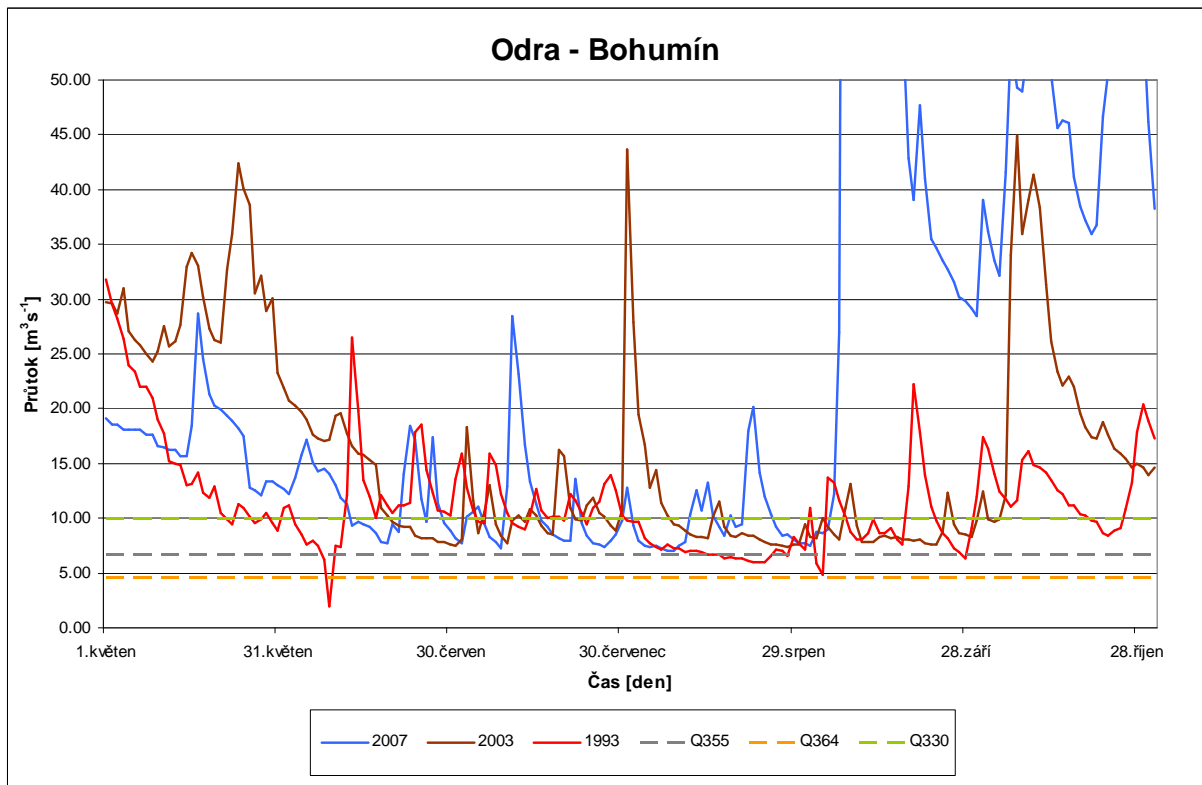
Hydrogramy vybraných povodňových událostí ve stanici Bohumín
