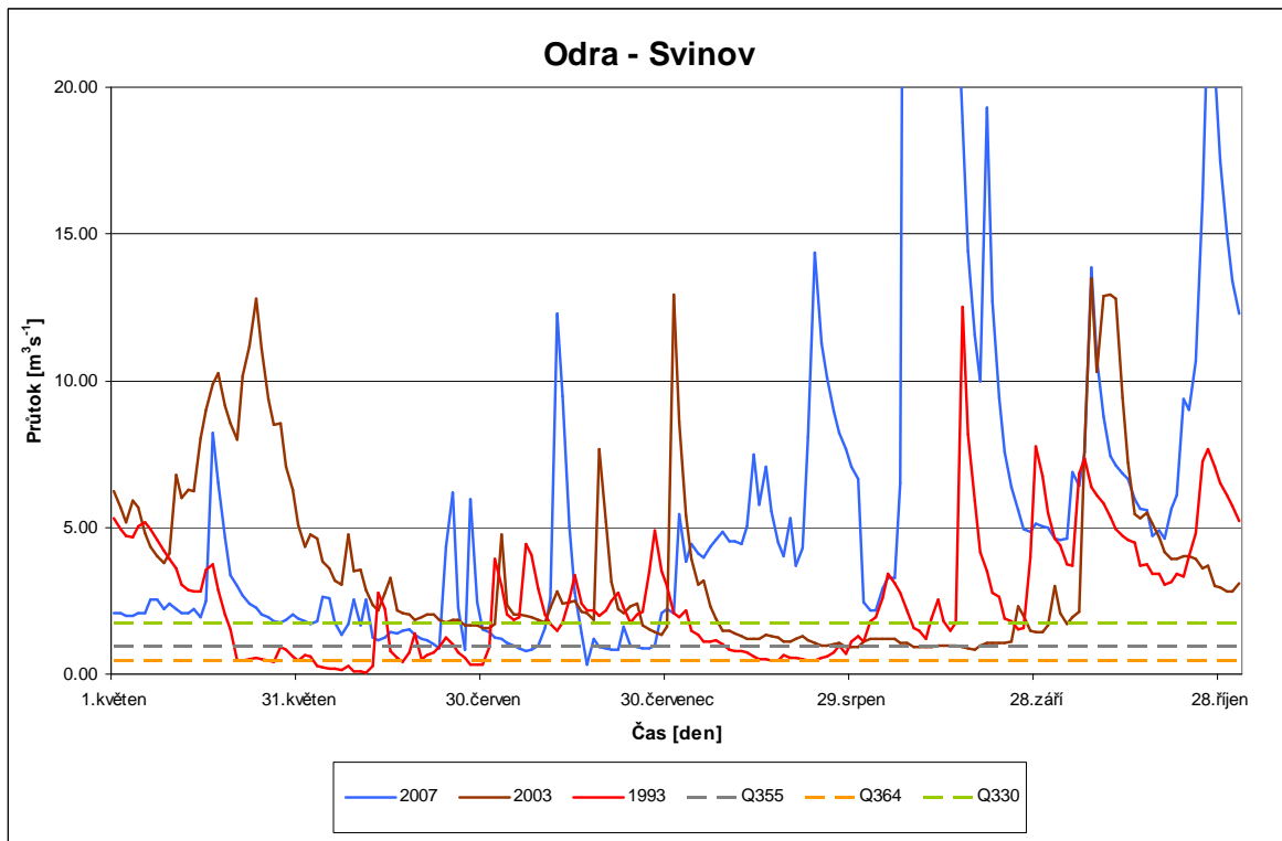
Hydrogramy vybraných povodňových událostí ve stanici Ostrava-Svinov
