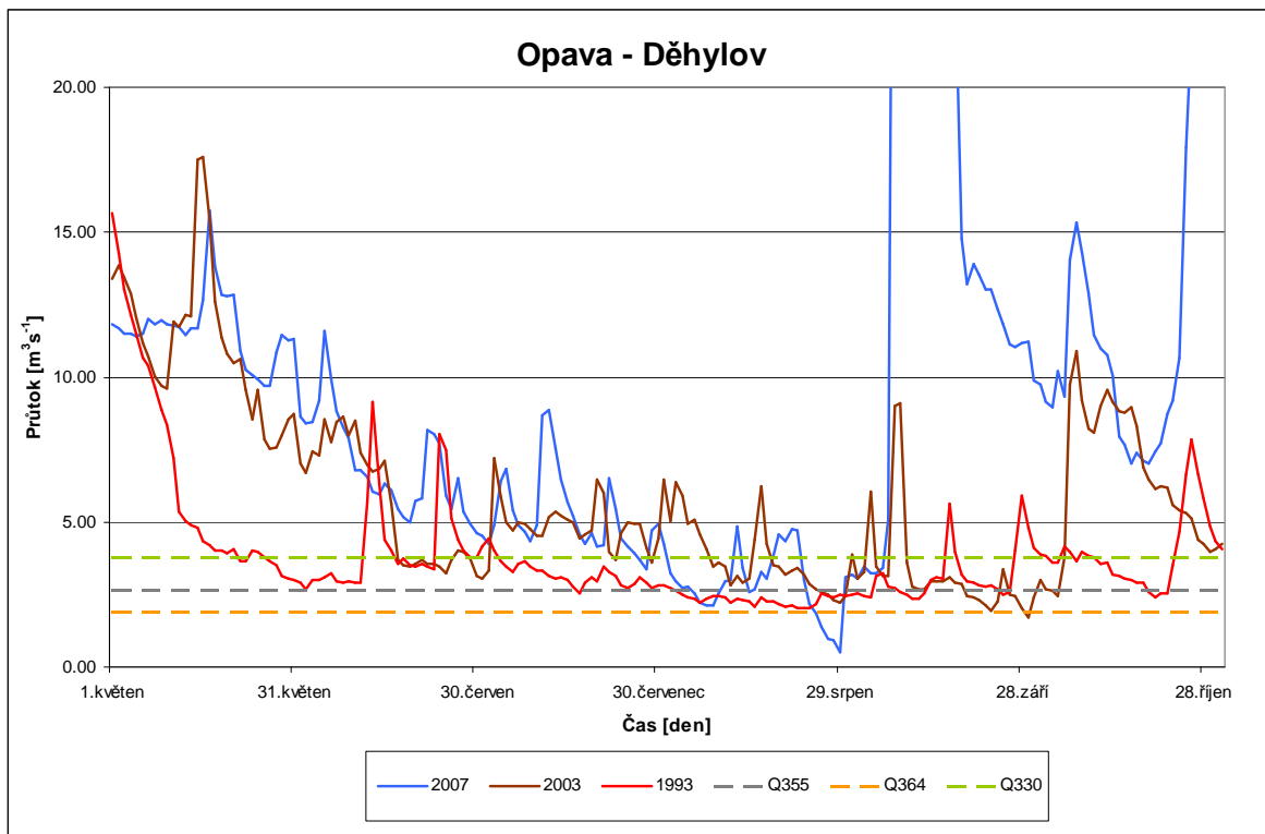
Hydrogramy vybraných povodňových událostí ve stanici Děhylov na řece Opavě
