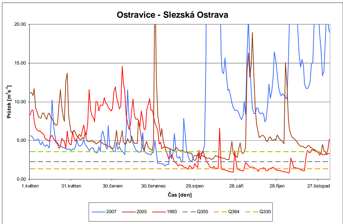
Hydrogramy vybraných povodňových událostí ve stanici Ostrava
